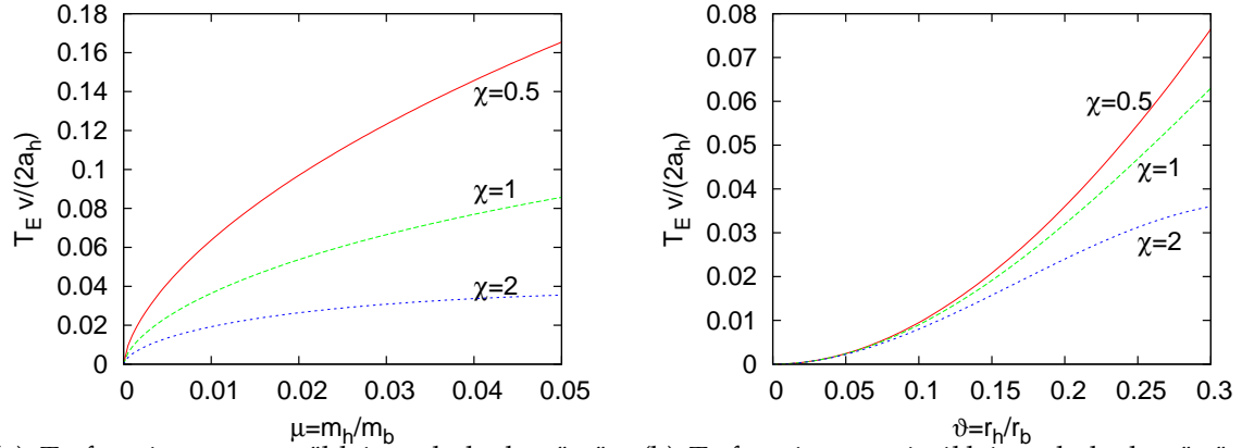
(a) T_E függése a tömegtől három különböző sűrűségarány esetén (b) T_E függése a sugártól három különböző sűrűségarány esetén
