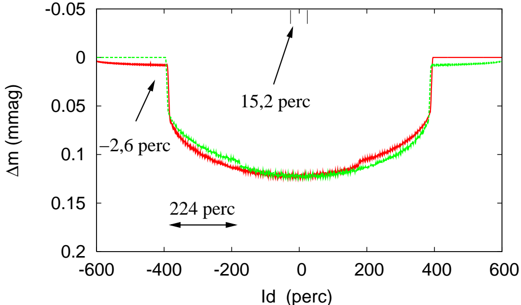
9. ábra. A Föld-Hold rendszer által generált fénygörbe pirossal vezető, zölddel követő hold esetén.
