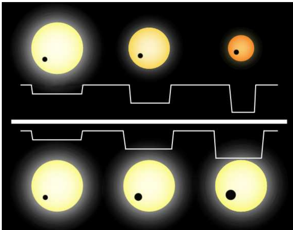
2. ábra. Fedések mélységének függése a hőmérséklettől, sugáraránytól.
