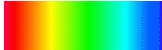
folytonos spektrum
